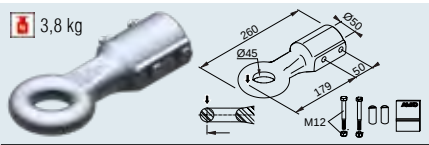
SAP: ZUGÖSE I45 M SCHRAUBMAT VZ Argolla para Italia I45/F N.º de ref. 1224108
