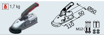
SAP: KUPLNG KUGL AK161 D50 M MONTTEILE Embrague AK 161 - Ø 50 N.º de ref. 1730808
