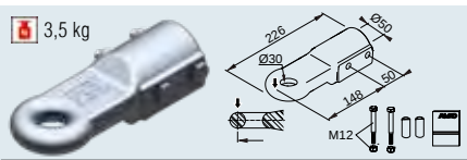
SAP: ZUGÖSE E30 M SCHRAUBMAT VZ Argolla para Inglaterra E30/A N.º de ref. 1224106
